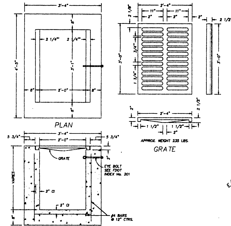
TYPE "C" INLET SCALE: 1/2" = 1'
