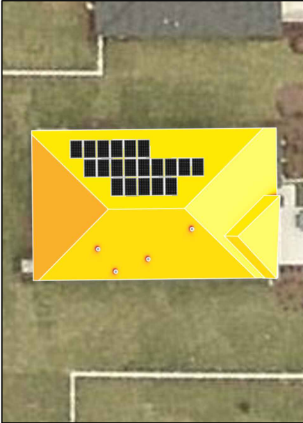
3 IRRADIANCE MAP N.T.S.
