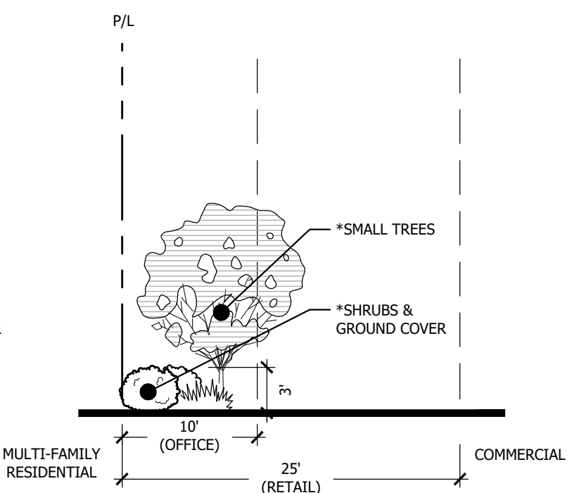
COMMERCIAL - LESS INTENSE USE BUFFER DETAIL SCALE: N.T.S.
